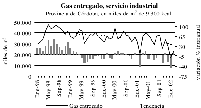
Fuente Ente Nacional Regulador del Gas, Enargas. Últimos datos disponibles a abril 2002.
