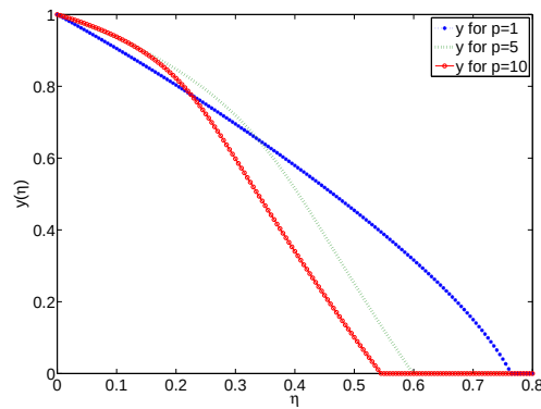
Figura 1: Gráfica de la función y para diferentes valores de p = 1, 5, 10 , fijando \delta = 5 y Ste = 0,5 .
