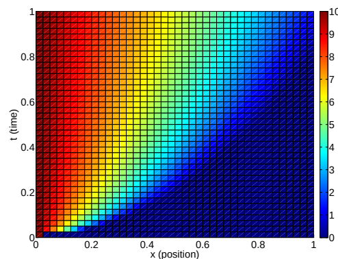
Figura 2: Mapa de colores para la función T = T(x, t) fijando \delta = 1 , p = 1 , Ste = 0,5 , T_f = 0 , T_0 = 10 y a = 1
